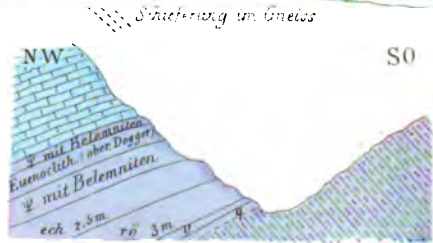
Fig. 10. Querprofil am Contact an der Orfluh (Meltenberg)
